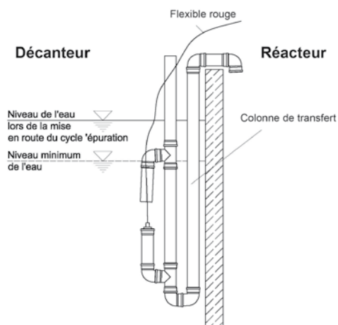
Colonne de transfert.
