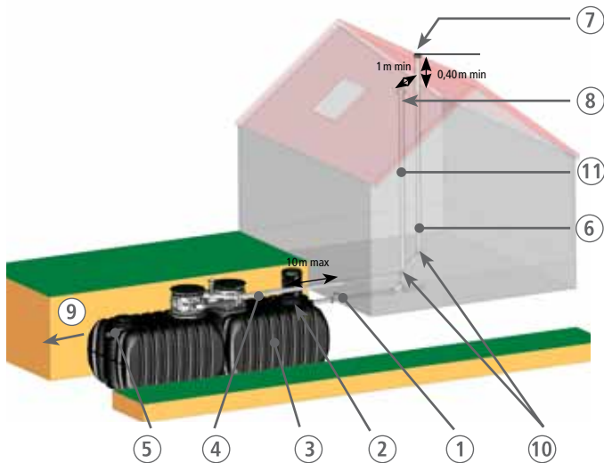
Schéma de raccordement de la ventilation haute pour une micro-station ACTIBLOC® 12EH (10000 QR).
