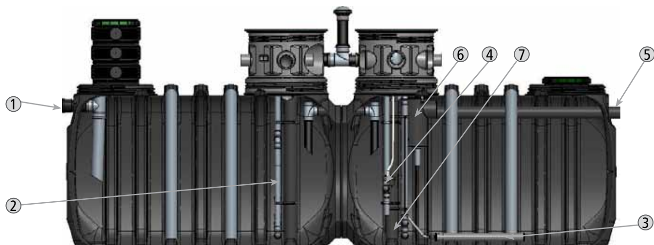
Vue de coupe d'une micro-station ACTIBLOC® 12EH (10000 QR).
